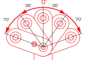
5段階 (35°) に可変可能なマルチパーパスバー
